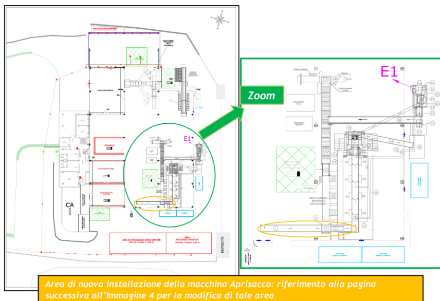
Figura 40: STRALCIO DEL LAYOUT ATTUALE CON INDIVIDUAZIONE DELL'AREA DI INSTALLAZIONE
