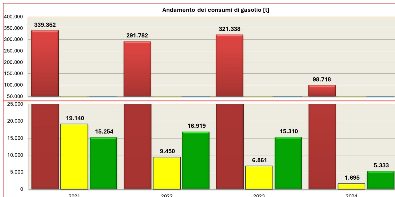
Figura 27: ANDAMENTO DEL CONSUMO DI GASOLIO ATTIVITÀ PRINCIPALI
