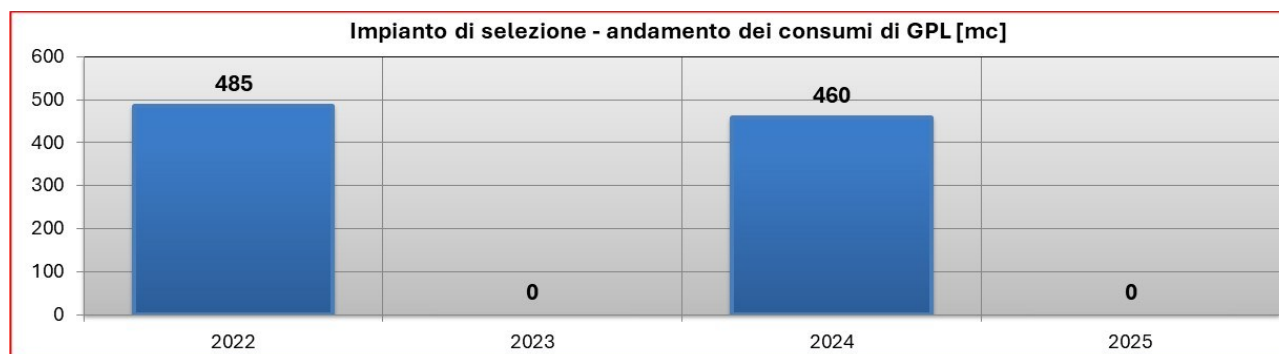
Figura 29: CONSUMO DI GPL PER RISCALDAMENTO SITO_3
