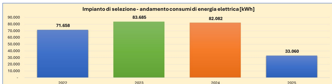
Figura 25: CONSUMI ENERGIA ELETTRICA SITO_3: IMPIANTO DI SELEZIONE
