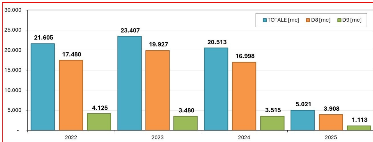
Figura 34: CONSUMO DI ACQUA SITO_2
