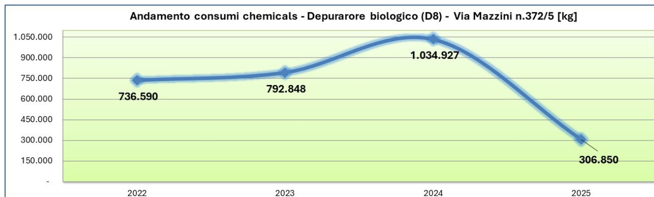
Figura 31: CONSUMO DI PRODOTTI CHIMICI - IMPIANTO D8
