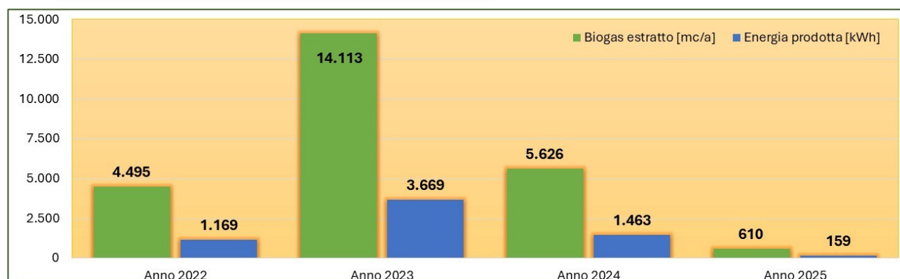
Figura 6: ANDAMENTO DEL BIOGAS ESTRATTO E DELLA ENERGIA ELETTRICA PRODOTTA
