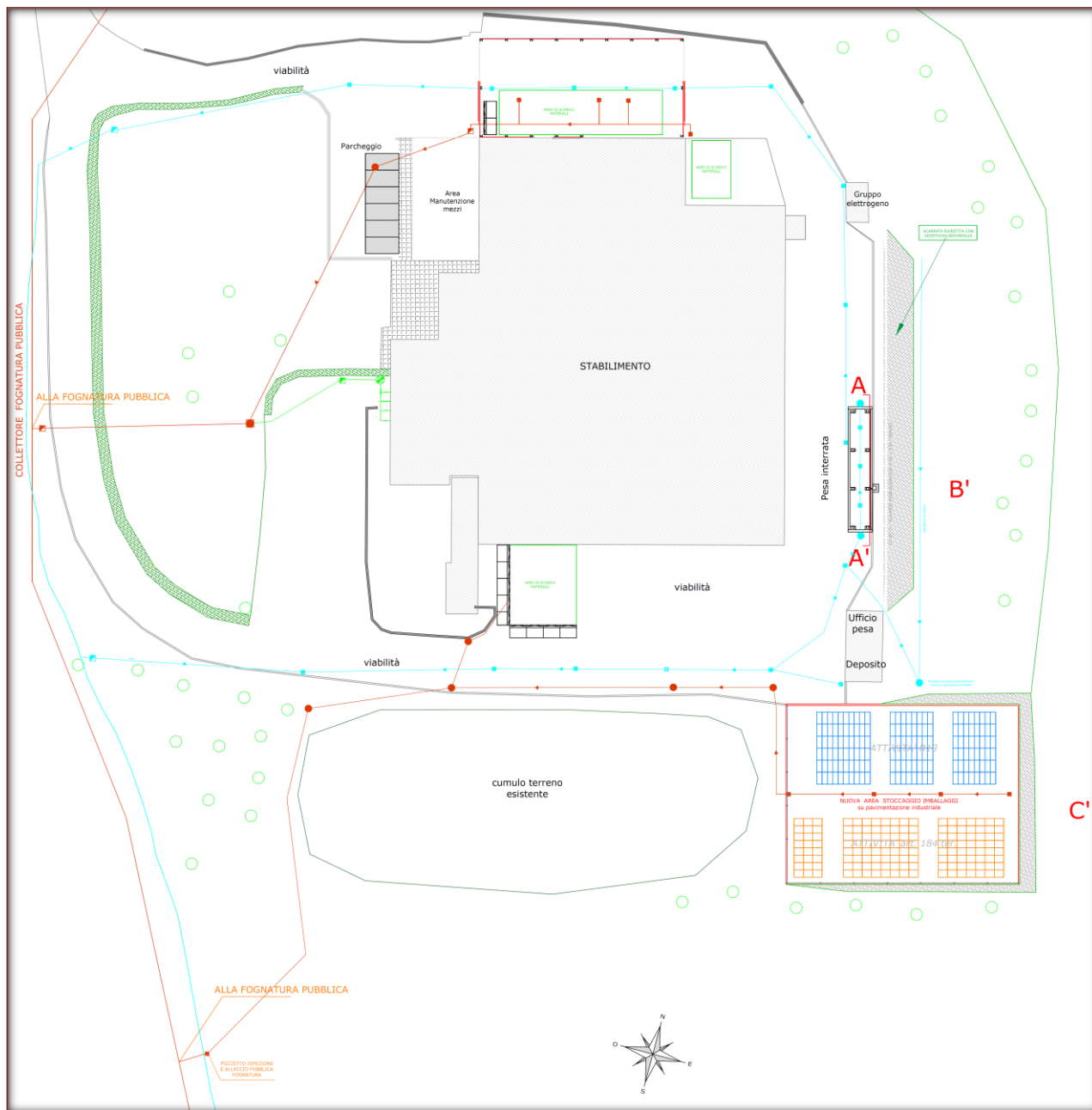
Figura 37: PLANIMETRIA RETE ACQUE – IMPIANTO DI SELEZIONE
