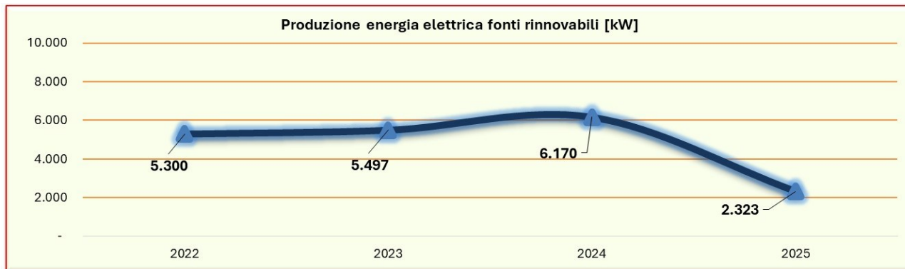
FIGURA 9: ANDAMENTO PRODUZIONE DI ENERGIA ELETTRICA DEGLI IMPIANTI FOTOVOLTAICI
