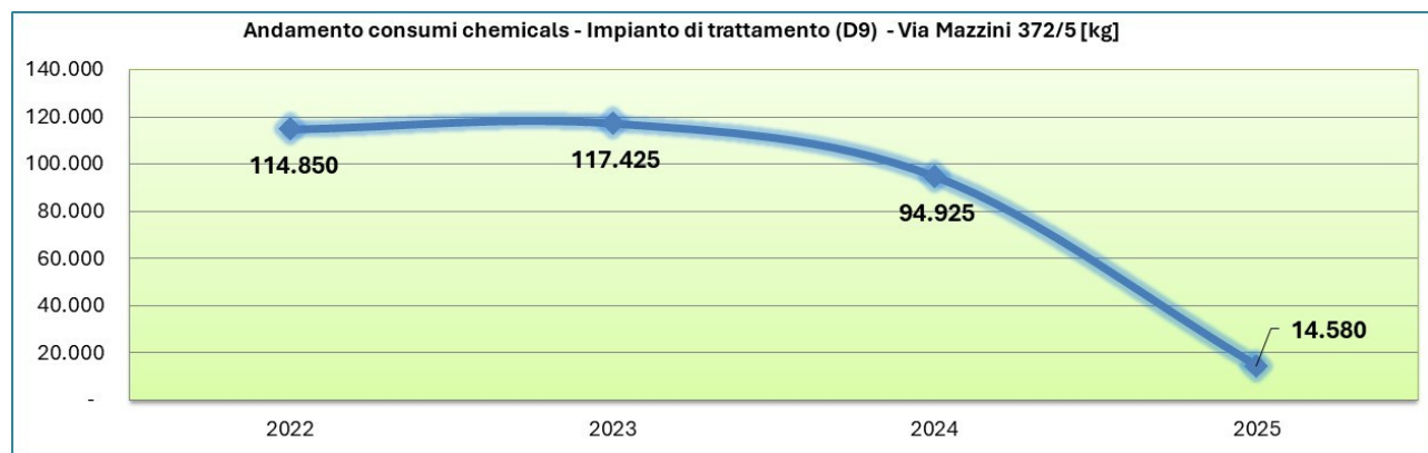
Figura 32: CONSUMO DI PRODOTTI CHIMICI – IMPIANTO D9
