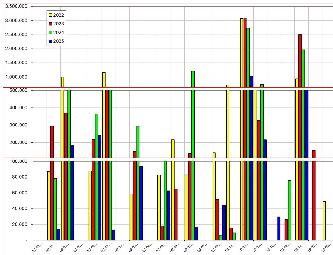
Figura 10: ANDAMENTO DEI RIFIUTI TRATTATI IN D8 SUDDIVISO PER CODICE CER
