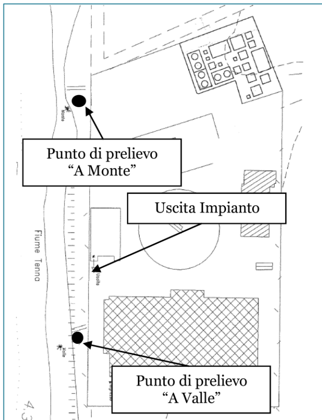
Figura 36: UBICAZIONE DEI PUNTI DI PRELIEVO
